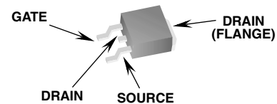
JEDEC TO-252AA
