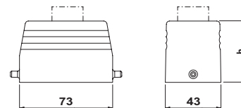
HC-B 10 TFL...
