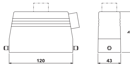
HC-B 24 TFL...
